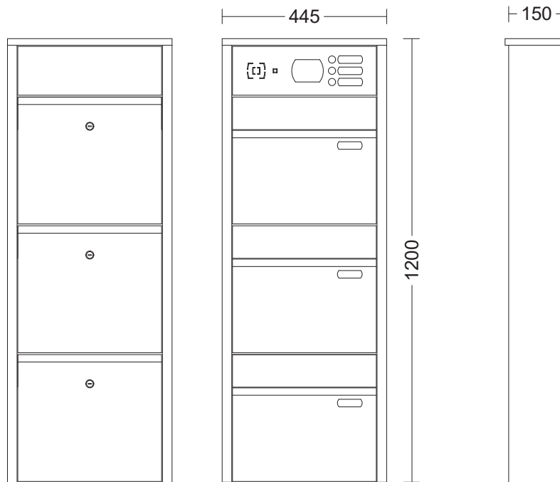
Rückansicht
