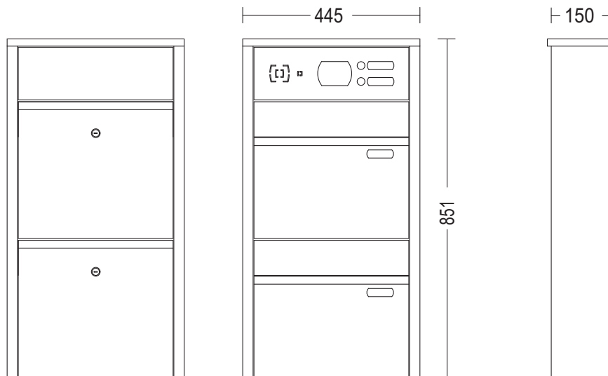
Rückansicht
