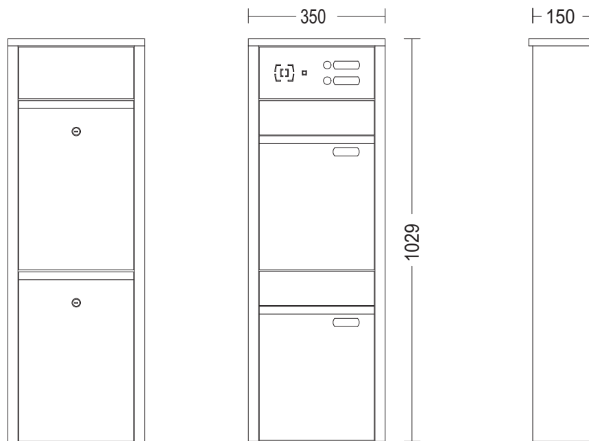
Rückansicht
