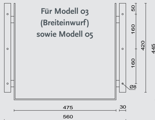
Art.Nr.: hd.03 B/05
