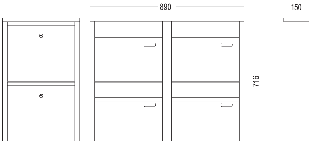
Rückansicht
